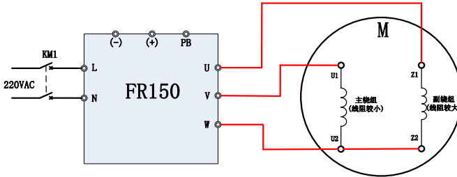
图 6-17 FR150A 与单相电机正转接线图
