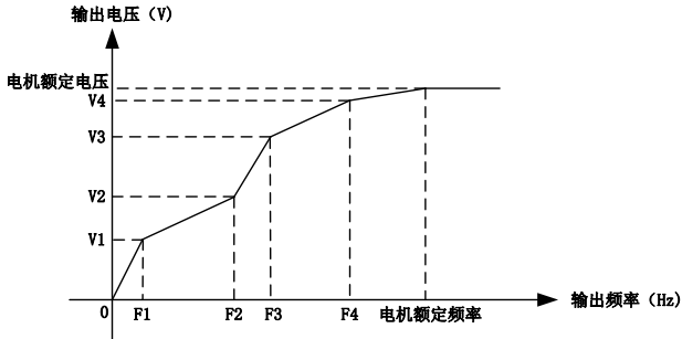
图 6-22 多点 VF 曲线示意图
