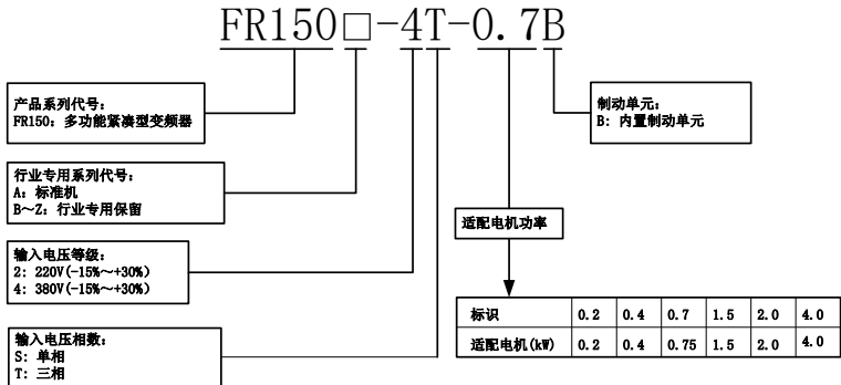
图 2-2 产品型号命名规则
