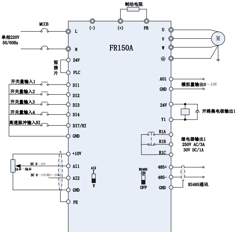
图 3-4a 单相 220V 变频器接线示意图 1 (<4.0kW)
