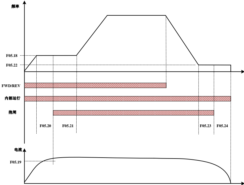
图 6-15 抱闸控制逻辑图
