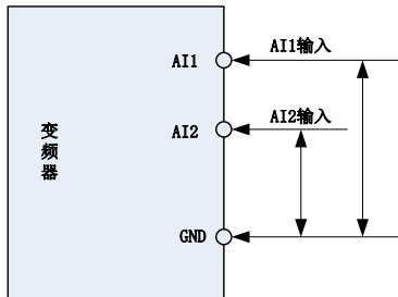
图 6-2 使用外部电源模拟量输入示意图
