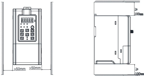
图 3-1 变频器安装示意
