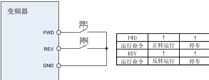
图 6-12 脉冲运行停车控制示意图
