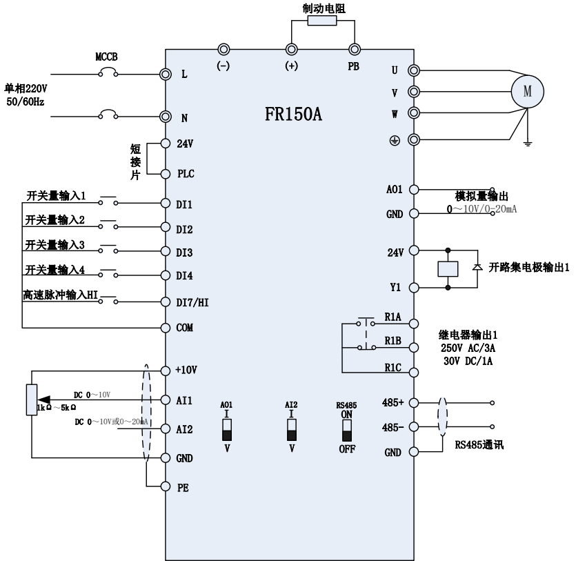
图 3-4b 单相 220V 变频器接线示意图 1 ( \geq 4.0\text{kW} )
