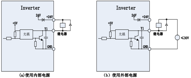
图 3-21 端子驱动继电器时的接线方式
