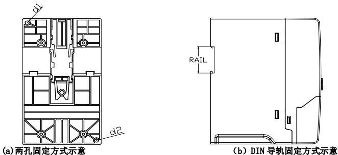
图 3-2 固定方式示意
