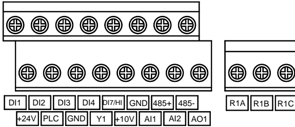
图 3-14 380 控制端子(&lt;5.5kW)或 220V 控制端子(&lt;4.0kW)示意图
