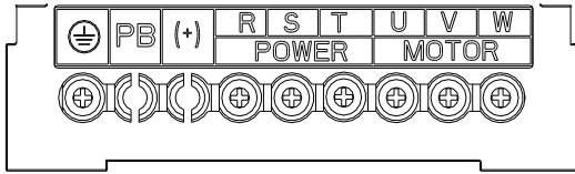
图 3-8 FR150A (0.7~4.0kW) 三相主回路端子
