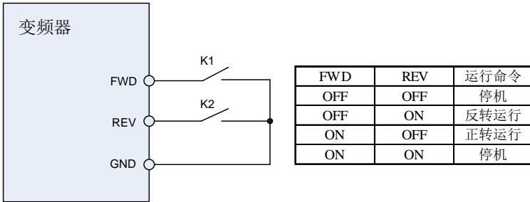
图 6-8 两线模式 1 控制示意图
