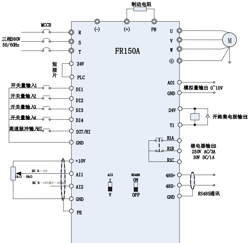
图 3-5a 三相 380V 变频器接线示意图 1 (<5.5kW)
