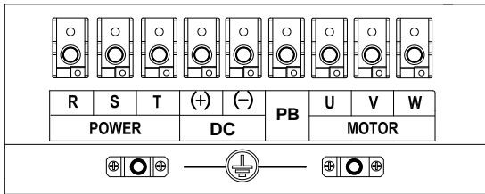
图 3-11 45~90kW 主回路端子示意图
