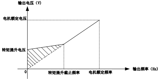
图 6-21 转矩提升示意图
