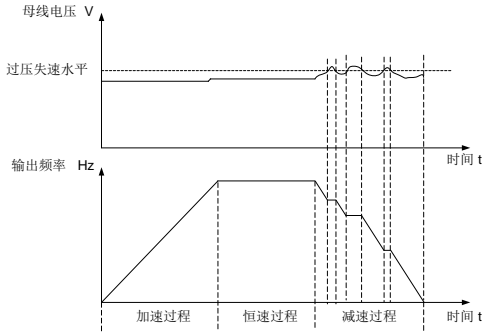
图 6-24 过压失速模式 1 示意图
