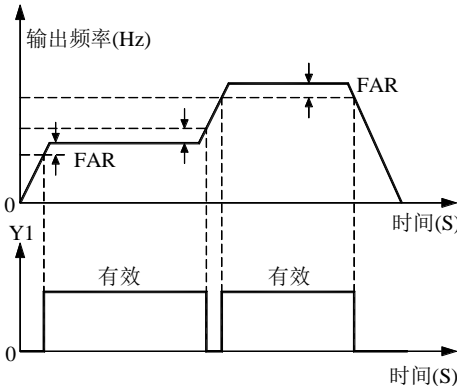
图 6-13 FAR 功能示意图
