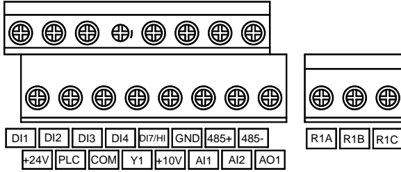
图 3-15 380 控制端子( \geq 5.5\text{kW} )或 220V 控制端子( \geq 4.0\text{kW} )示意图
