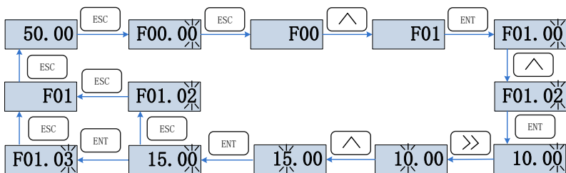
图 4-3 三级菜单操作举例
