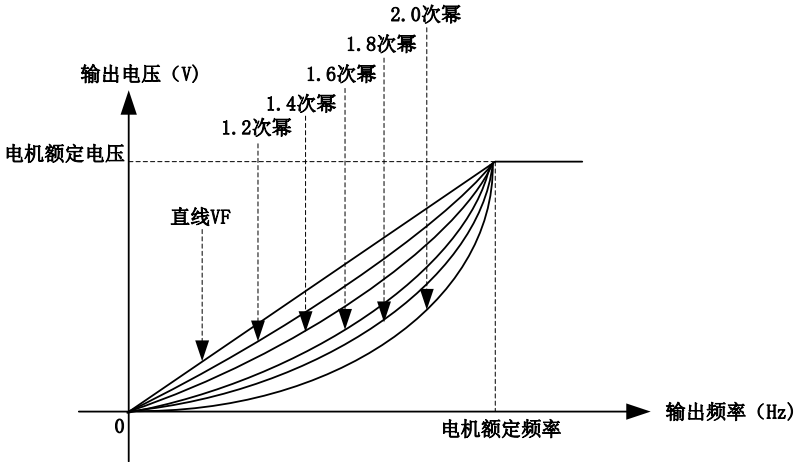
图 6-20 V/f 曲线示意图
