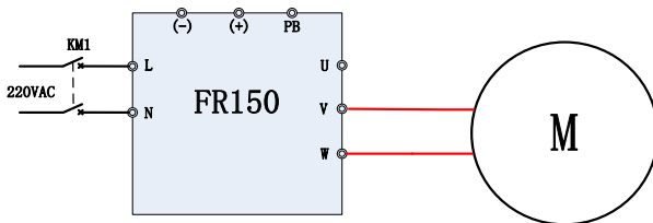
图 6-19 FR150A 与单相电机接线图
