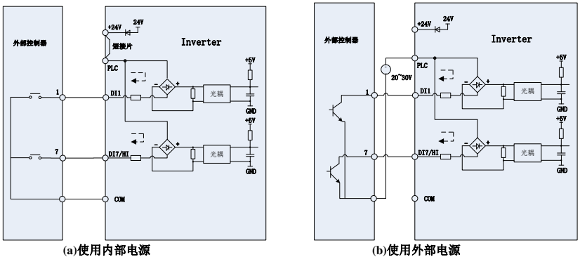
图 3-17 干接点方式
