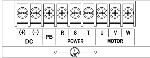
图 3-10 30~37kW 主回路端子示意图
