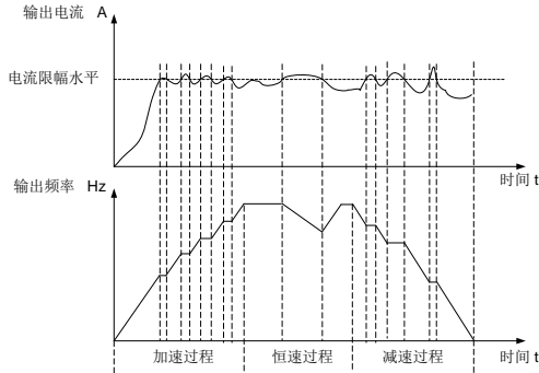
图 6-23 电流限幅模式 1 示意图
