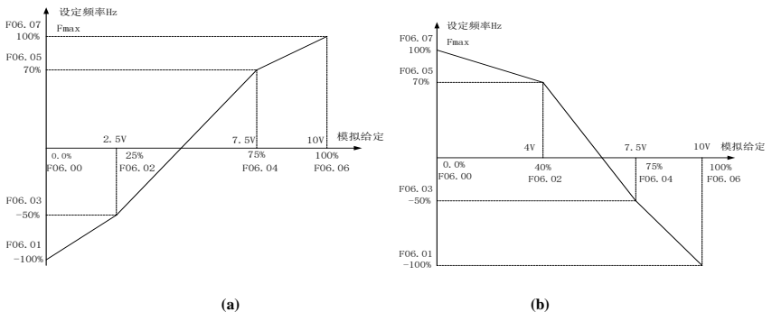
图 6-16 代码参数设定示意图
