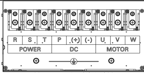
图 3-13 160kW 主回路端子示意图
