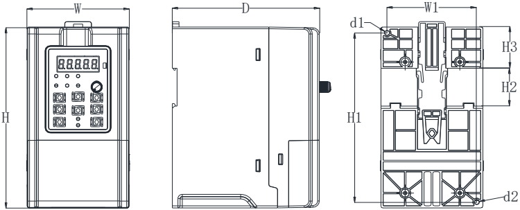
图 1-2 FR150A (0.2~22kW)产品尺寸示意图
