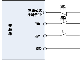
图 6-11 三线模式 2 控制示意图
