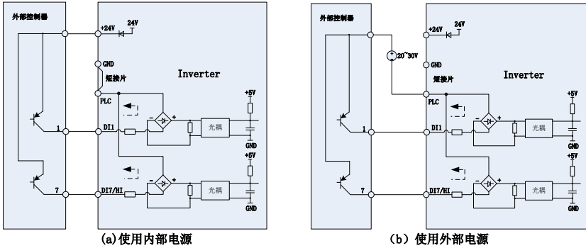
图 3-19 开路集电极 PNP 接线方式
