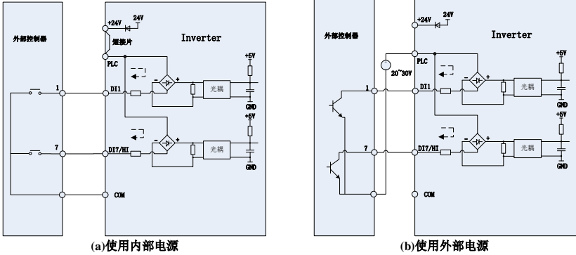
图 3-18 开路集电极 NPN 接线方式
