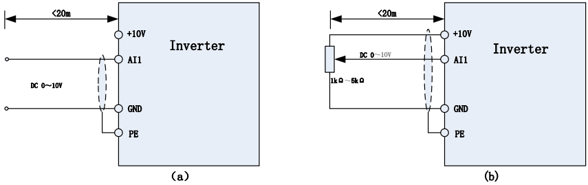
图 3-16 模拟量输入端子接线示意图
