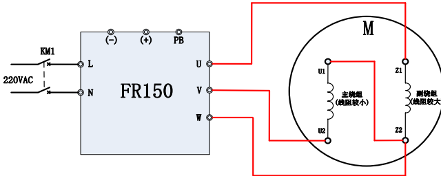
图 6-18 FR150A 与单相电机反转接线图
