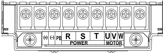
图 3-7 4.0kW 单相主回路端子示意图
