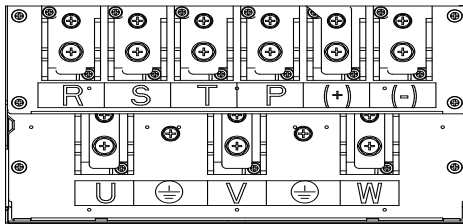
图 3-12 110~132kW 主回路端子示意图
