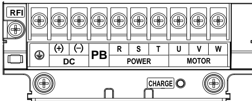
图 3-10 11~22kW 主回路端子示意图
