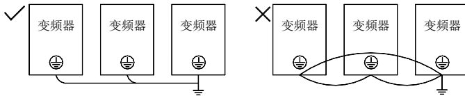
图 3-15 变频器接地处理
