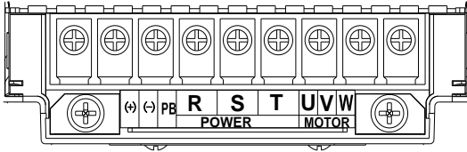
图 3-9 5.5~7.5kW 主回路端子示意图
