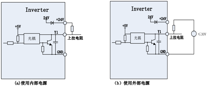
图 3-20 端子接上拉电阻输出时的接线方式
