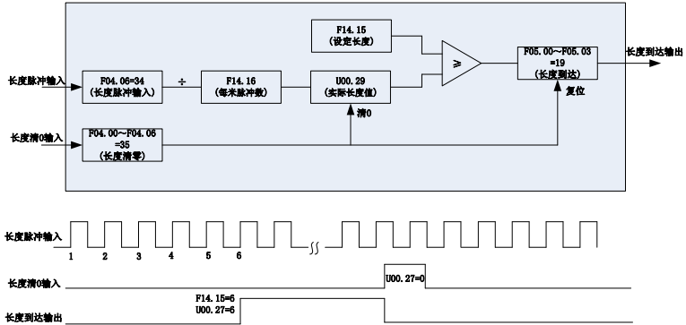
图 6-31 定长功能示意图
