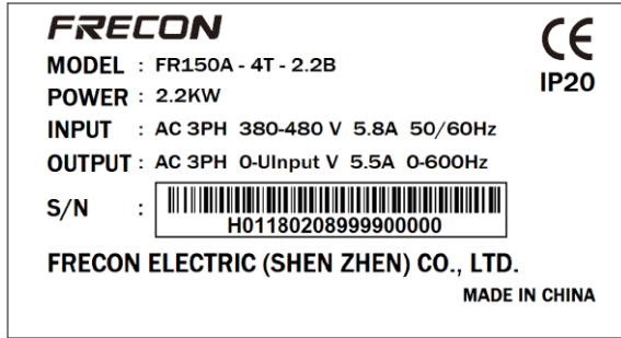
图 2-1 产品铭牌
