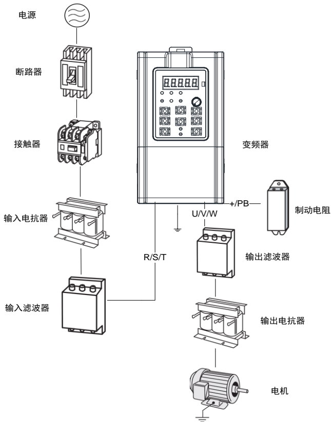
图 3-3 产品外围器件及配线
