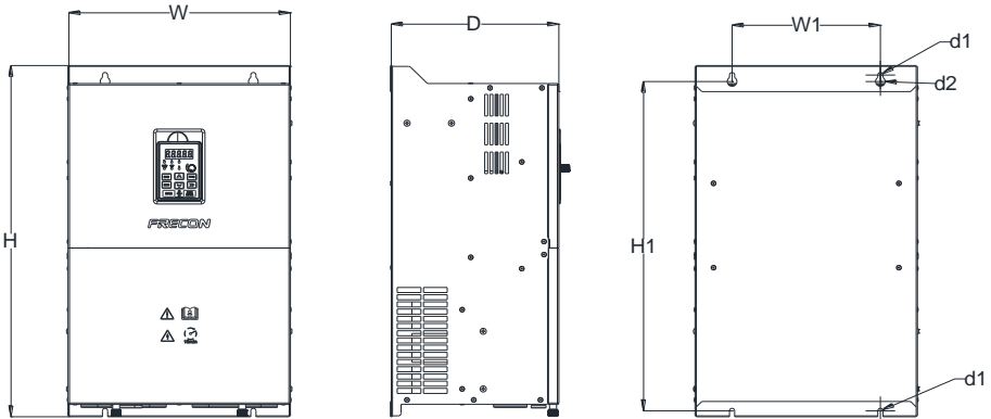
图 1-3 FR150A (30~160kW)产品尺寸示意图
