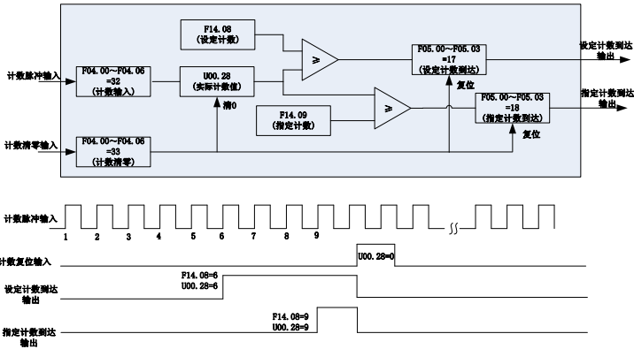
图 6-32 计数功能示意图
