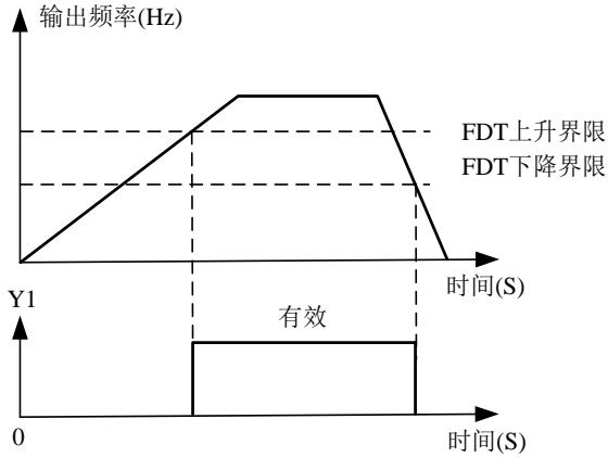
图 6-14 FDT 功能示意图
