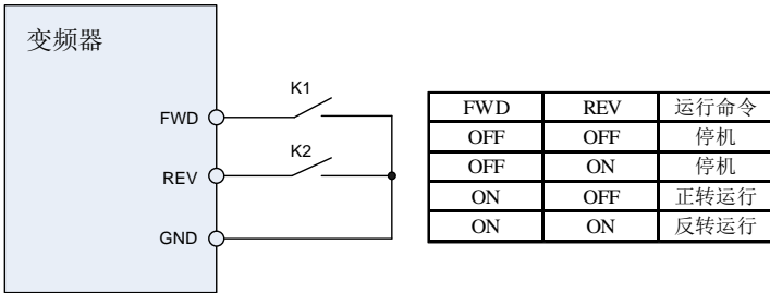
图 6-9 两线模式 2 控制示意图
